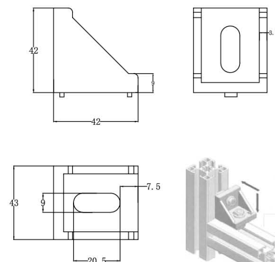
角件连接安装图
