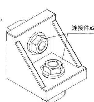
角件连接安装图
