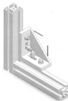
角件连接安装图
