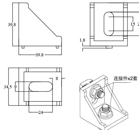
角件连接安装图
