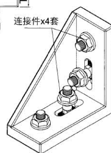
角件连接安装图
