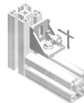
角件连接安装图
